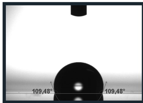
Formowanie się kropeł wody na lakierze z powłoką Ceramic Guard SiCarbon+ Coating
