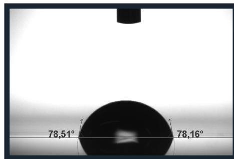
Formowanie się kropeł wody na lakierze bez powłoki Ceramic Guard SiCarbon+ Coating
